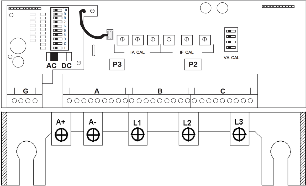
图 30 590C/35A—180A 电枢及三相输入端子
